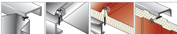
Esempi di installazione per fissaggi / Installation examples for fixings: AFM - AFM-RAINBOW - AFMX
